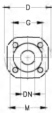
ФЛАНЦЫ НАСОСА
