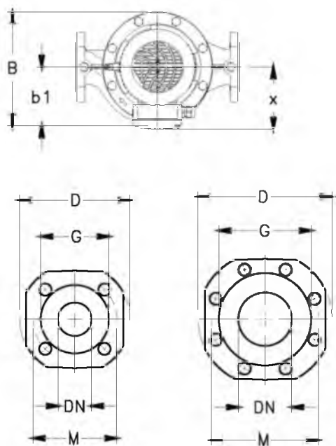
ФЛАНЦЫ НАСОСА
