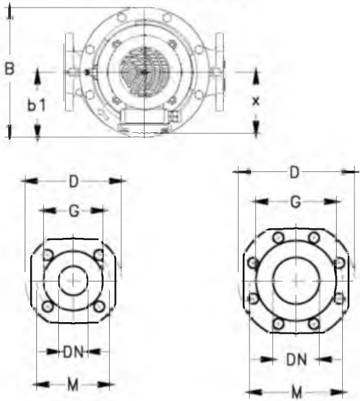
ФЛАНЦЫ НАСОСА
